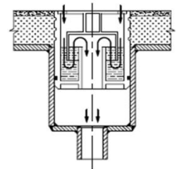
MONTAJE TÍPICO TYPICAL ASSEMBLY
