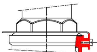
Seguro de tapa/ Locking bonnet
